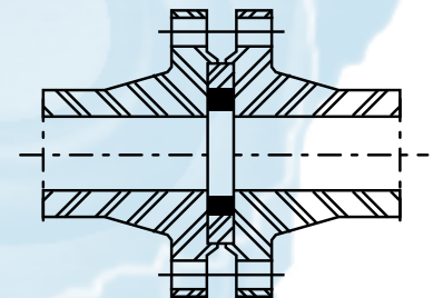
Vedação de flanges
