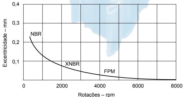
Excentricidade admissível aos eixos
