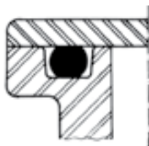
Deformação axial
