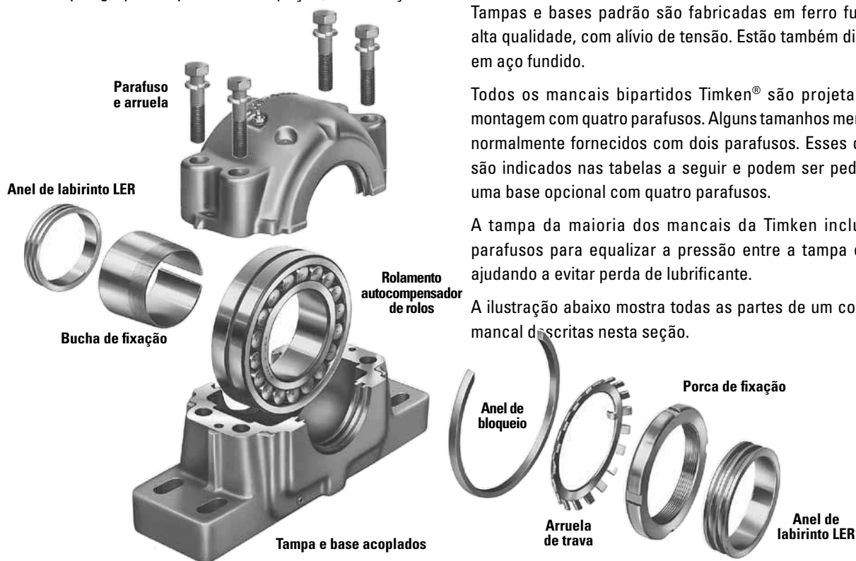
Fig. 26. Vista explodida de um mancal completo de rolamento autocompensador de rolos Timken, mostrando rolamento autocompensador de rolos de furo cônico, bucha de fixação, porca de fixação e arruela de trava, anel de bloqueio e retentores de labirinto triplos. São mostrados também os rebaixos na tampa e na base que formam o entalhe para ferramenta extratora, e asas do pedestal na base e na tampa.
