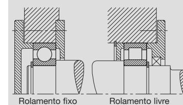
Rolamento fixo Rolamento livre
