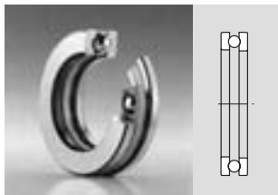
Rolamento axial de esferas escora simples
