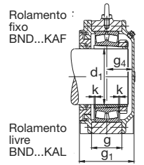
Execução A
