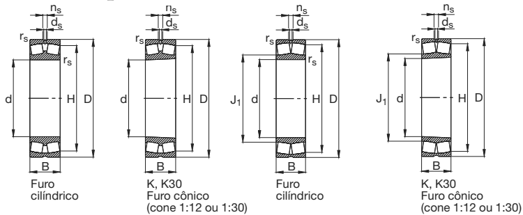
Construção E
