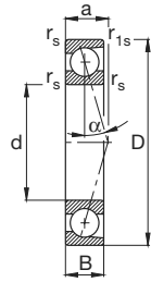
B719C, B70C Ângulo de contato \alpha = 15^\circ
