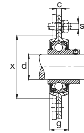
FB2 combinado com 362
