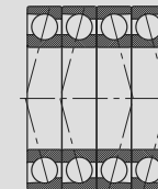
QBC Disposição em O
