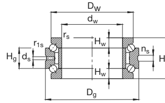
2344, 2347 Ângulo de contato \alpha = 60^\circ
