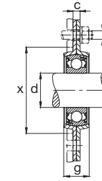
FB2 combinado com 562
