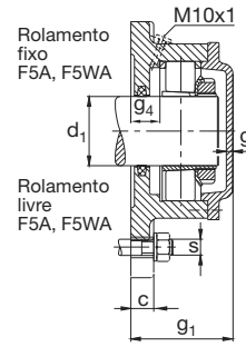
Execução A
