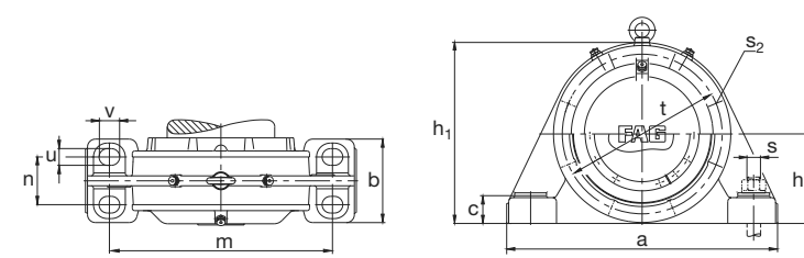
Para os cortes transversais das caixas BND para rolamentos com furo cilíndrico vide à página 663
