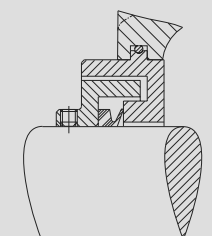
Vedações combinadas de labirinto + vedação de contato (Taconite)
