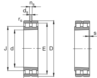
NN30ASK (conicidade 1:12)
